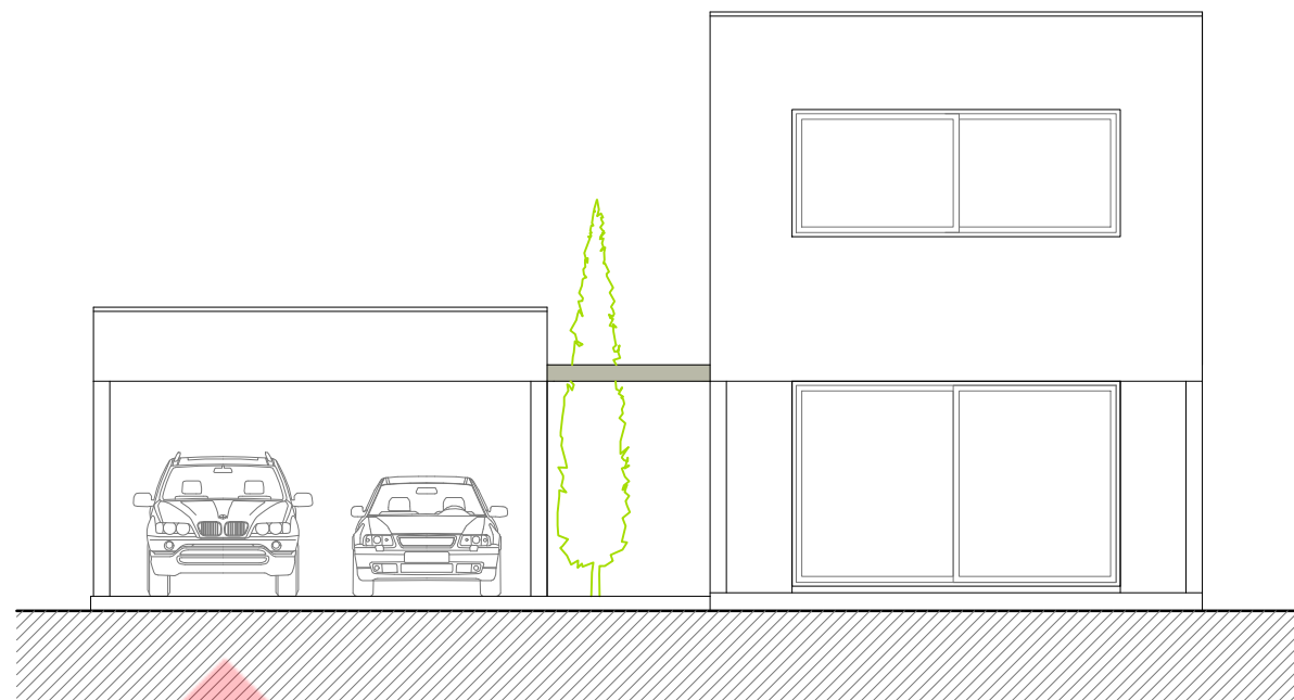
FAÇANA POSTERIOR
